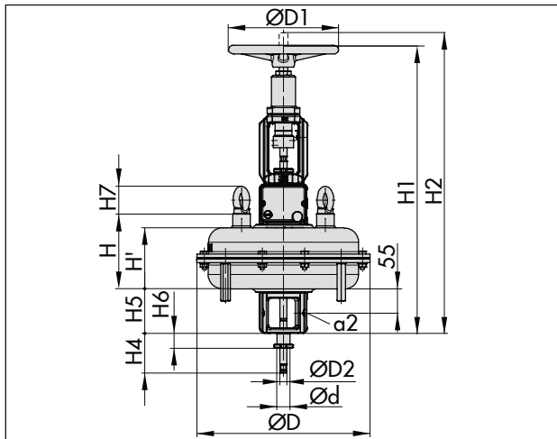
Fig. 26 : Type 3277 avec limitation de course des deux côtés et commande manuelle
