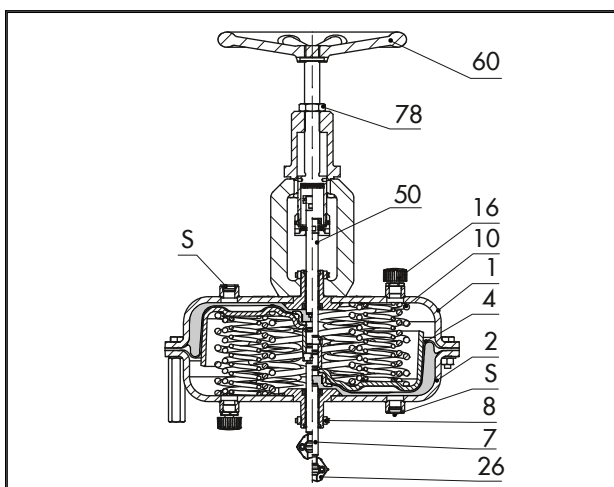
Fig. 11 : Type 3271 avec commande manuelle supplémentaire (exemple de représentation avec surface de 750v2 cm 2 )
