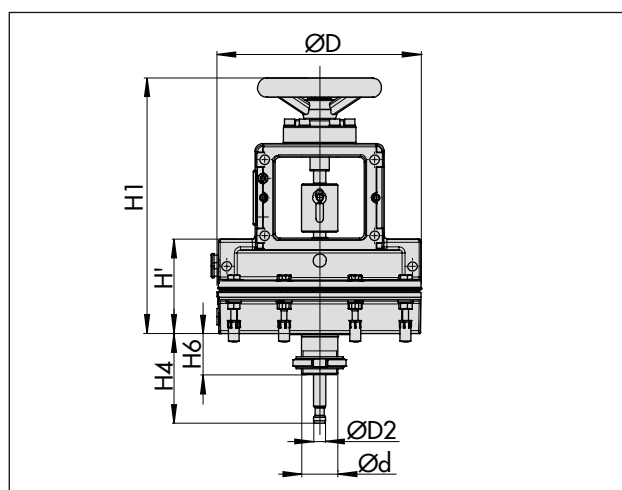
Fig. 16 : Type 3271-5 avec commande manuelle supplémentaire
