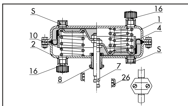
Fig. 7 : Type 3271 · Moitié droite avec ressorts supplémentaires
