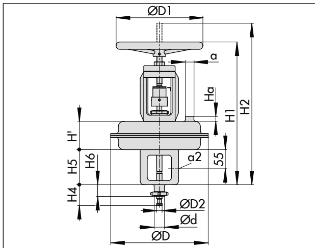
Fig. 25 : Type 3277 avec commande manuelle supplémentaire
