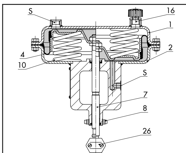
Fig. 9 : Type 3277 pour le montage direct d'accessoires (exemple de représentation avec surface de 350 cm 2 )
