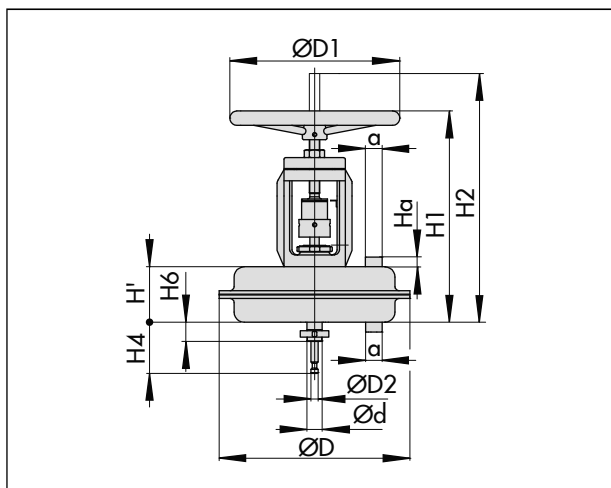
Fig. 18 : Type 3271 avec commande manuelle supplémentaire
