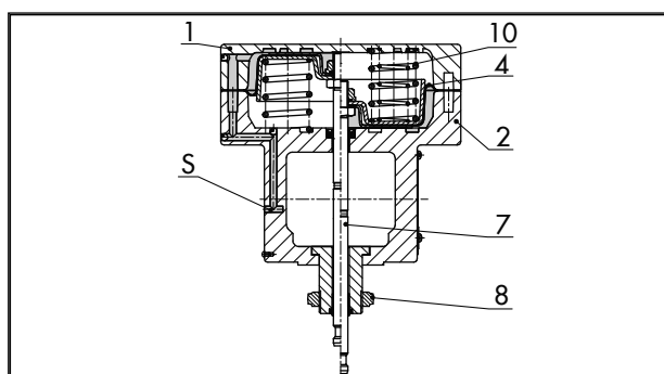
Fig. 8 : Type 3277-5 pour le montage direct d'accessoires (120 cm 2 )
