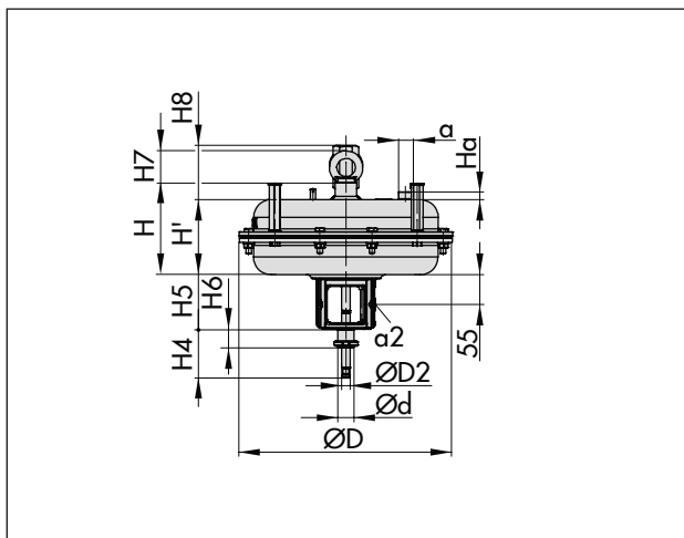
Fig. 27 : Type 3277 avec limitation de course
