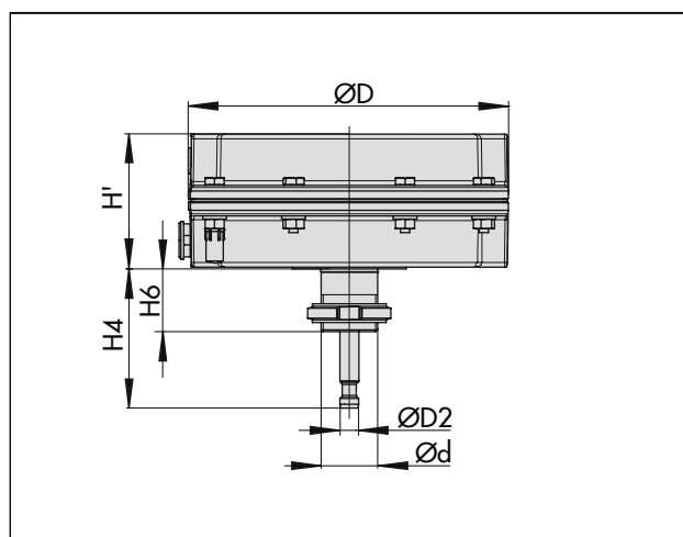
Fig. 15 : Type 3271-5 · Surface du servomoteur 120 cm 2
