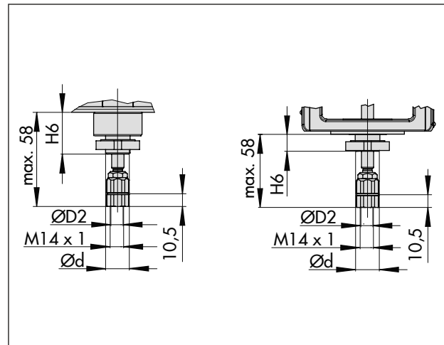
Fig. 28 : Type 3271-5 et type 3277-5 avec course de 7,5 mm pour vanne microdébit type 3510
