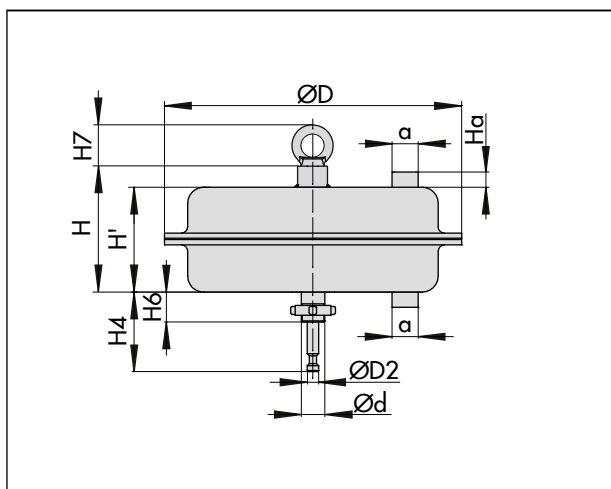
Fig. 17 : Type 3271 avec surface de 750v2 cm 2
