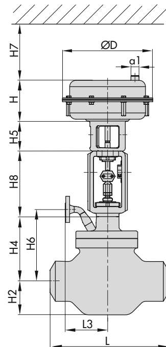
Typ 3281-7 mit Anschweißenden
