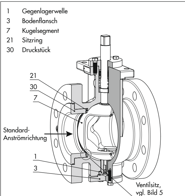
Bild 3: Kugelsegmentventil Typ 3310
