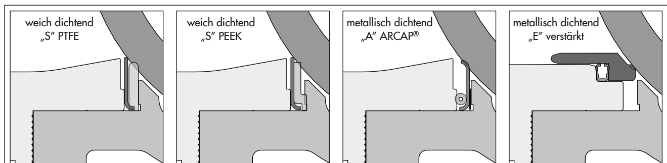
Bild 5: Ventilsitze
