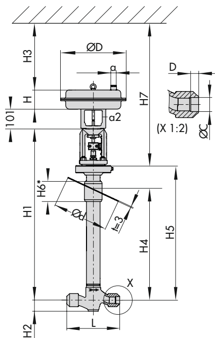
Bild 6: Durchgangsventil Typ 3248-7
