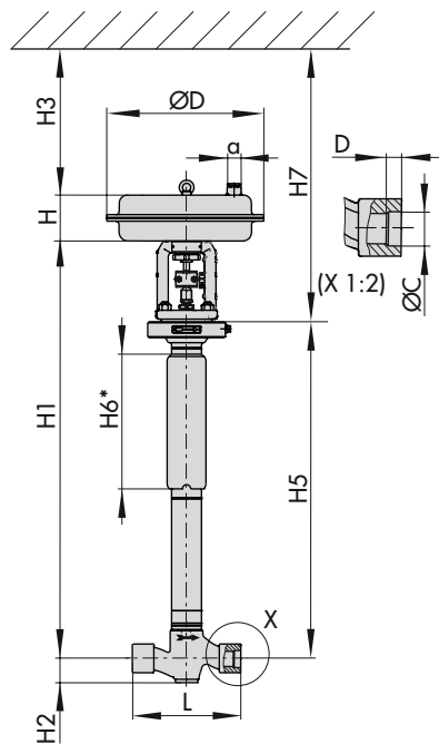
Bild 5: Durchgangsventil Typ 3248-1
