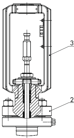
Bild 3: Oberteil und Joch für Class 600
