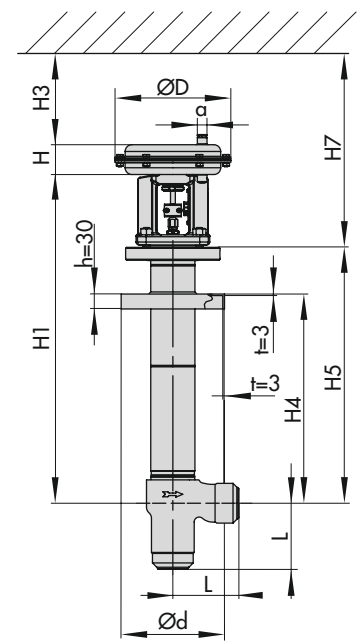
Bild 7: Eckventil Typ 3248-1
