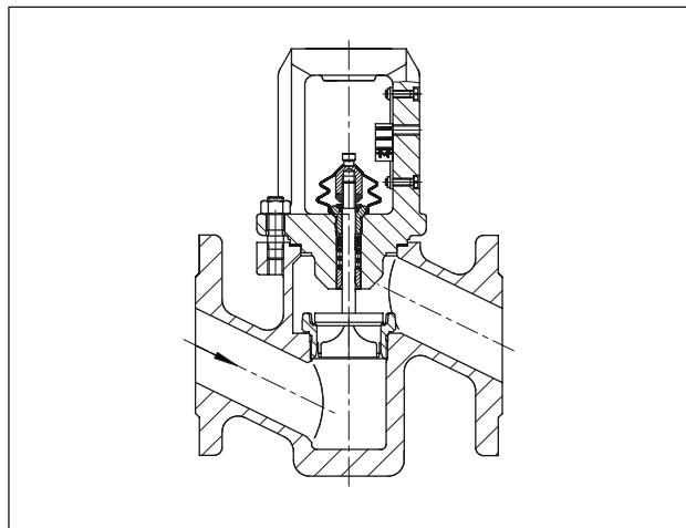
Fig. 2: Valvola Tipo 3241 PSA · Versione in acciaio forgiato · DN 15 fino a 80
