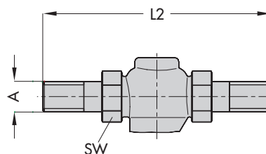
Ausführung mit Verschraubungen und Anschraubenden
