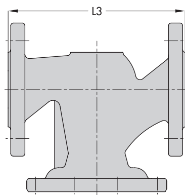
Ausführung mit Flanschgehäuse
