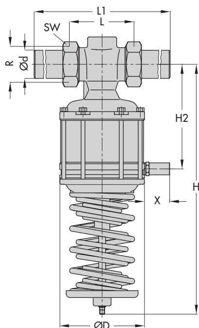
Ausführung mit Verschraubungen und Anschweißenden
