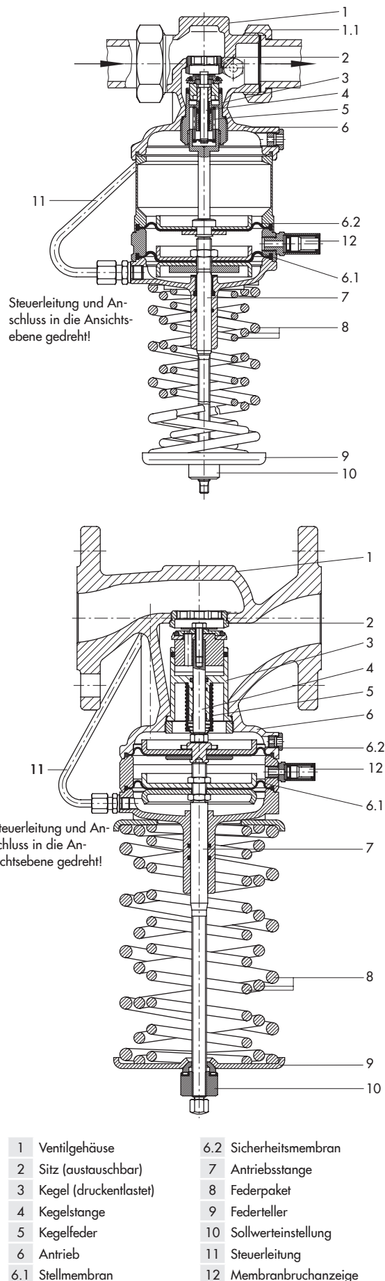
Bild 3: Wirkungsweise, Gehäuse mit Gewindeanschluss und Flansch
