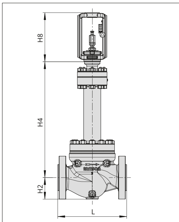
Bild 16: Ventil Typ 251GR mit Balgteil
