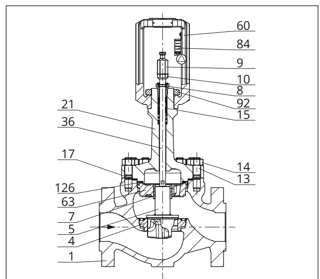
Bild 5: Ventil Typ 251GR mit Isolierteil
