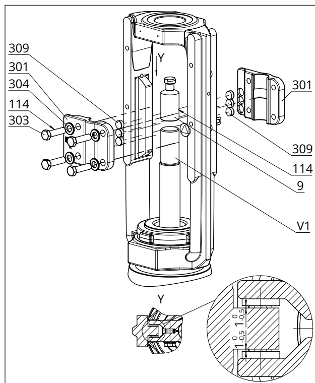
Bild 23: Montageübersicht der Verdrehssicherung in der Standardausführung
