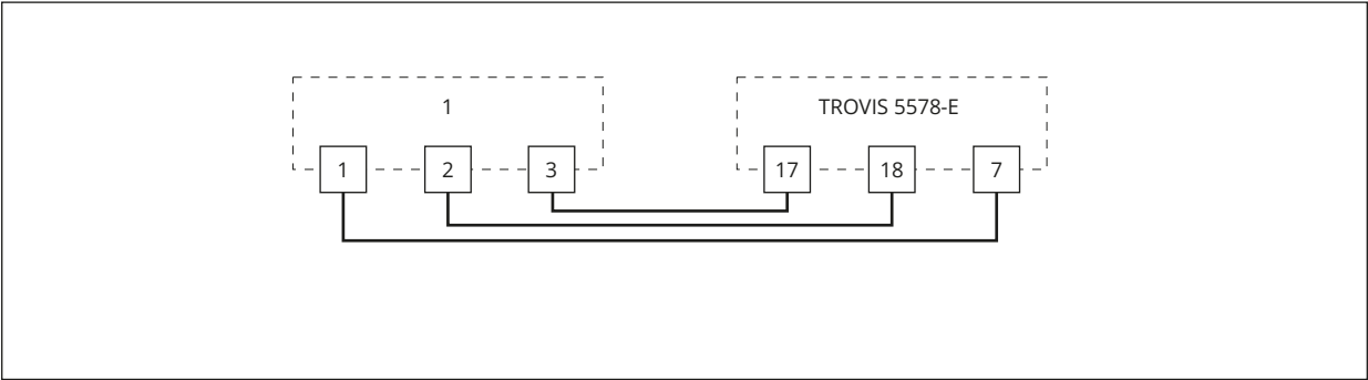
Bild 7: Anschluss eines Raumleitgeräts für RK3
