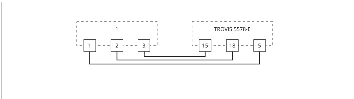
Bild 5: Anschluss eines Raumleitgeräts für RK1
