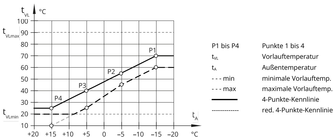
Bild 16: 4-Punkte-Kennlinie
