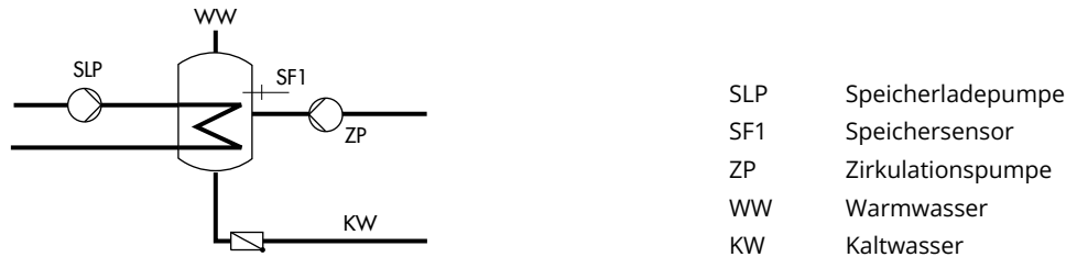
Bild 17: Aufbau eines Speichersystems
