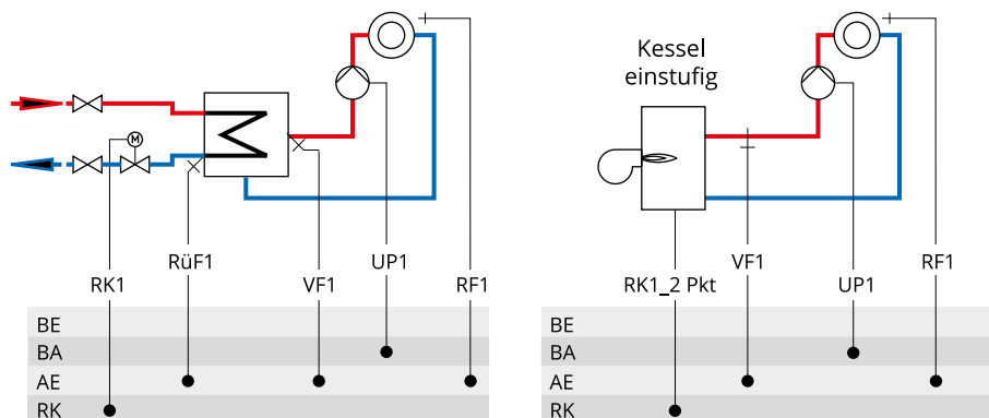
Bild 14: Konzipierung einer Kesselanlage
