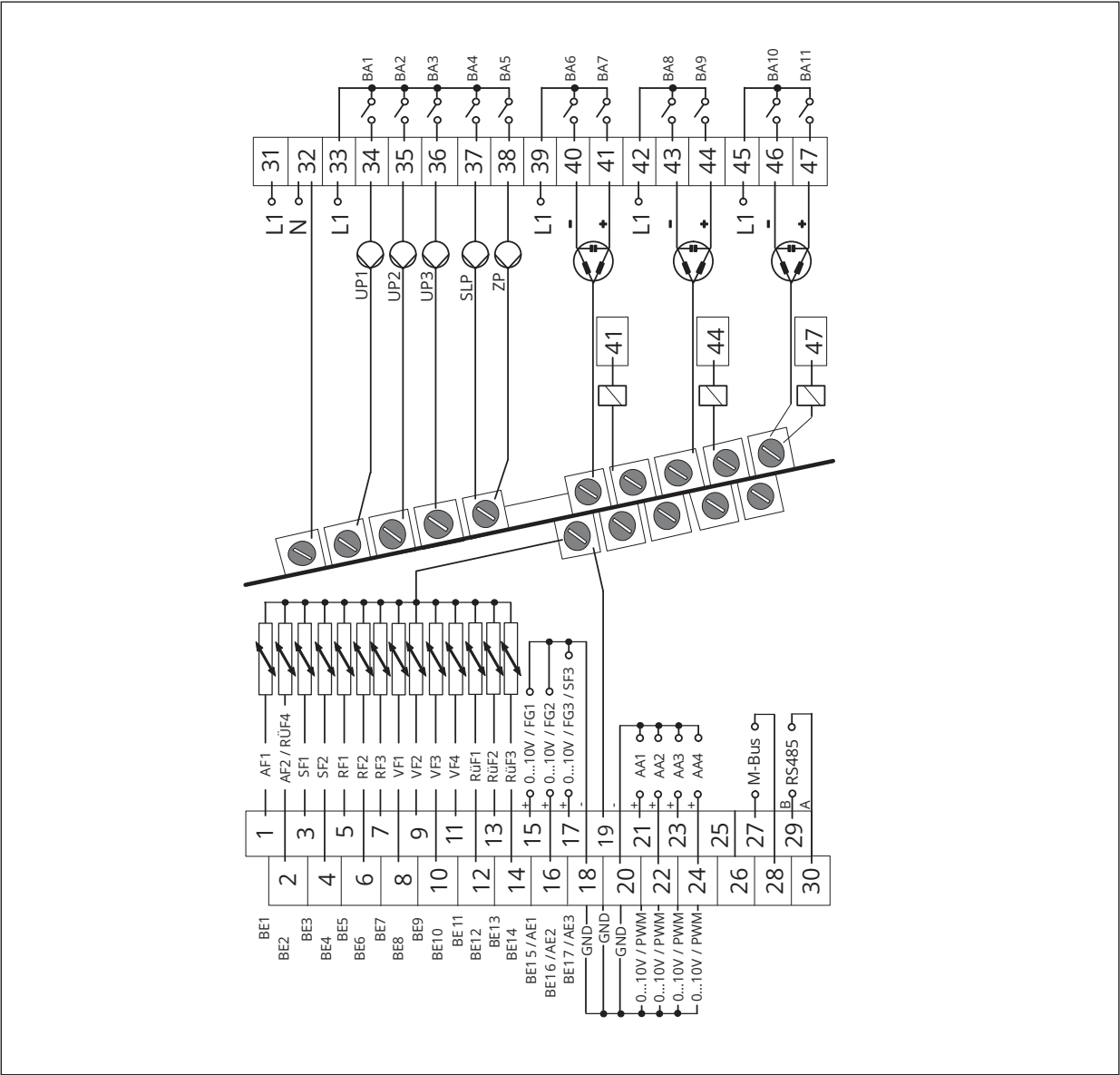
Bild 3: Elektrischer Anschluss TROVIS 5578-1113
