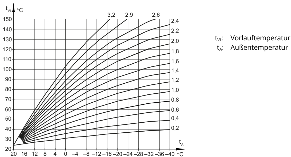
Bild 15: Steigungskennlinien
