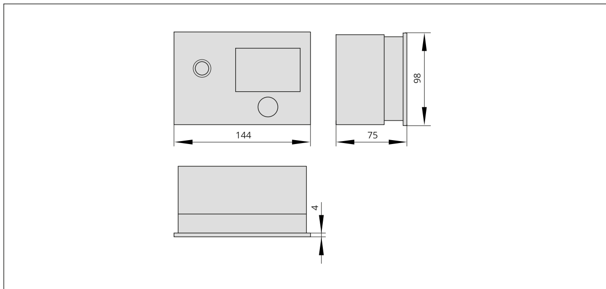
Bild 1: Maße in mm · Heizungs- und Fernheizungsregler
