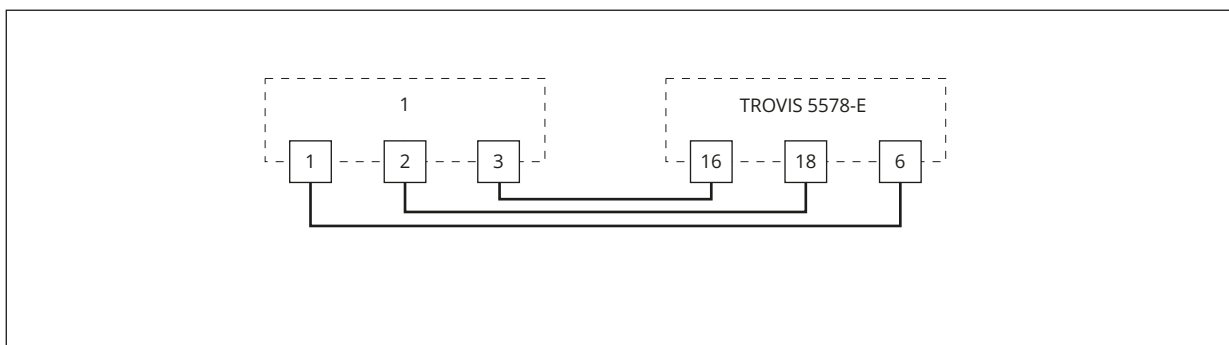
Bild 6: Anschluss eines Raumleitgeräts für RK2
