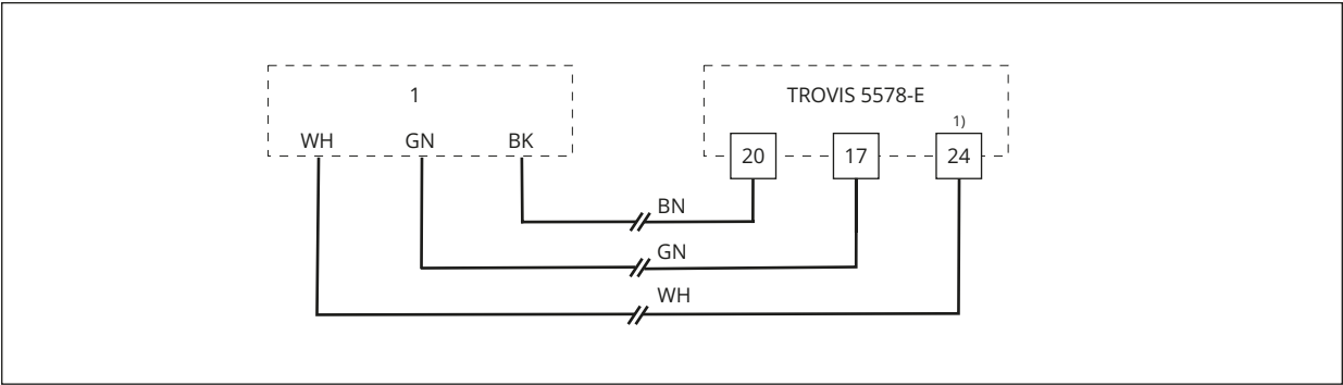
Bild 8: Anschluss eines Wasserströmungssensors
