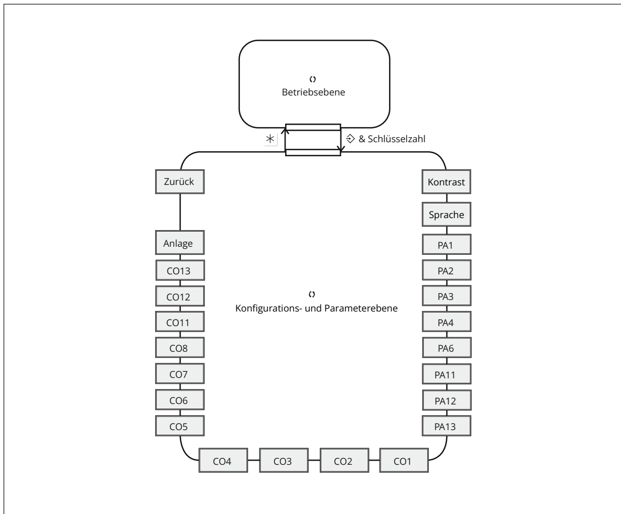
Bild 10: Ebenenstruktur TROVIS 5578-E
