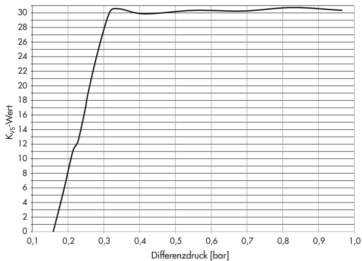
DIN Ventilkennlinie und Durchflusstabelle für DN 50 · K_{vs} 32
