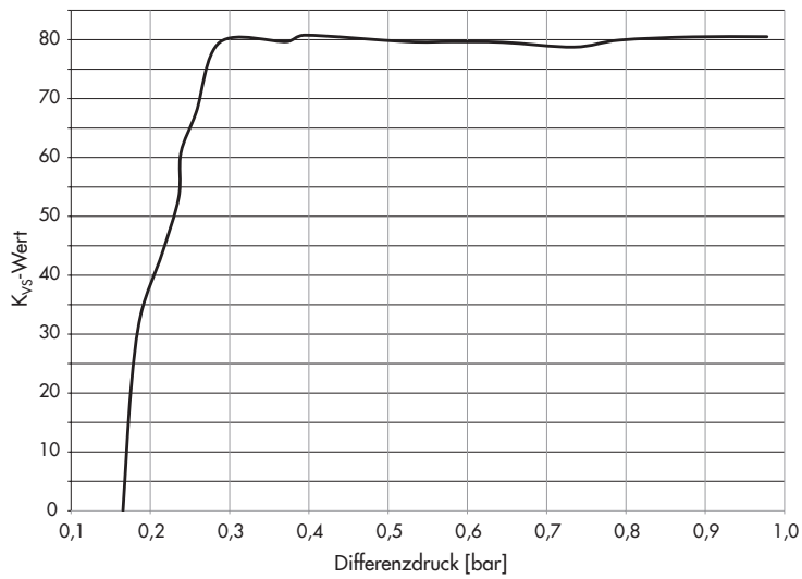
DIN Ventilkennlinie und Durchflusstabelle für DN 80 · K_{vs} 80
