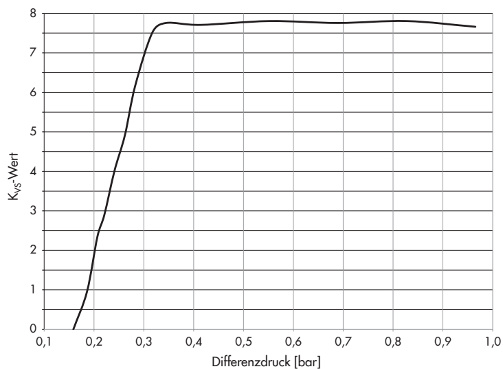
DIN Ventilkennlinie und Durchflusstabelle für DN 25 · K_{VS} 8
