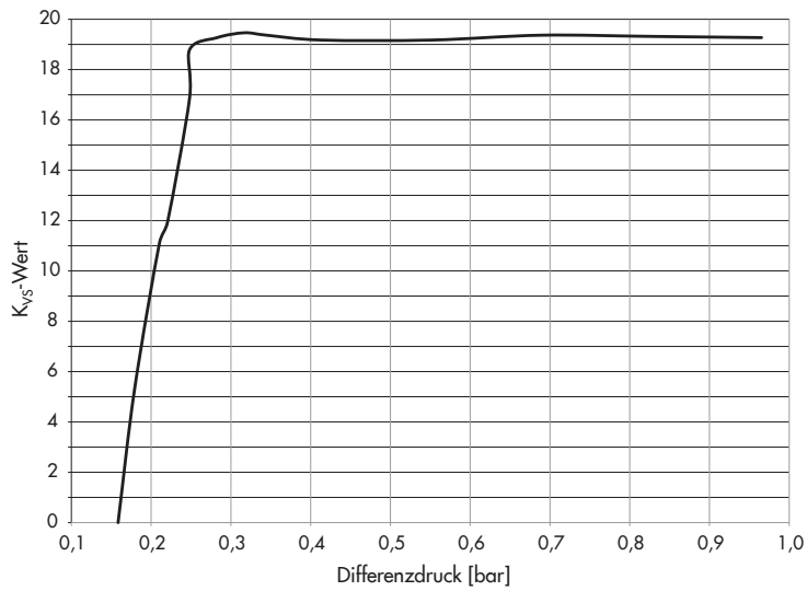
DIN Ventilkennlinie und Durchflusstabelle für DN 40 · K_{vs} 20
