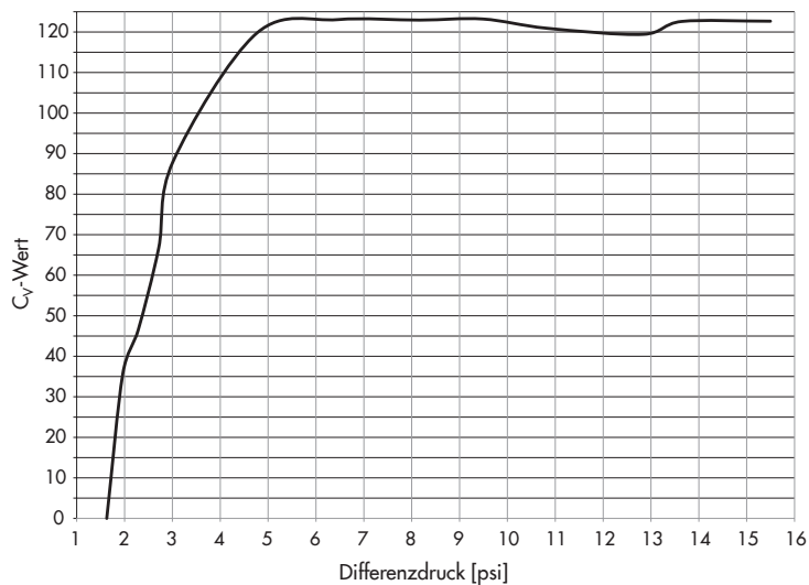
Bild 7-7: Ventilkennlinie und Durchflusstabelle für DN 100/NPS 4
