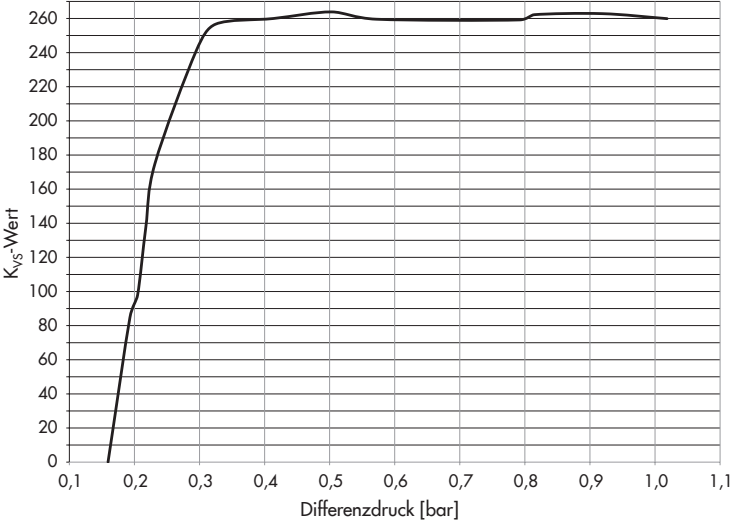
DIN Ventilkennlinie und Durchflusstabelle für DN 150 · K_{VS} 280
