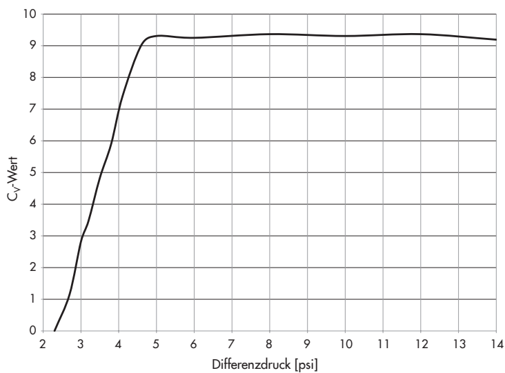
Bild 7-3: Ventilkennlinie und Durchflusstabelle für DN 25/NPS 1
