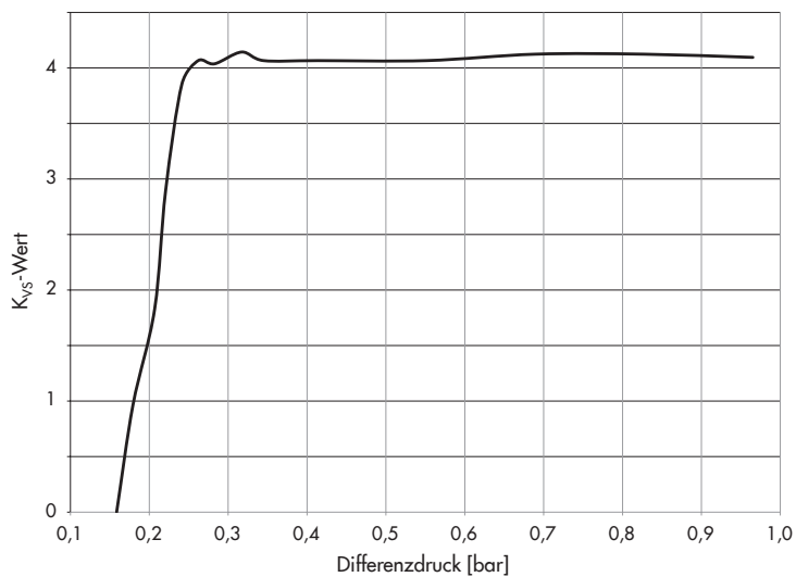
DIN Ventilkennlinie und Durchflusstabelle für DN 15 · K_{vs} 4
