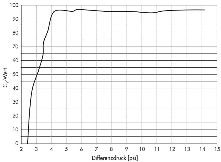
Bild 7-6: Ventilkennlinie und Durchflusstabelle für DN 80/NPS 3
