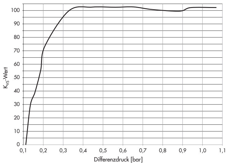
DIN Ventilkennlinie und Durchflusstabelle für DN 100 · K_{vs} 125
