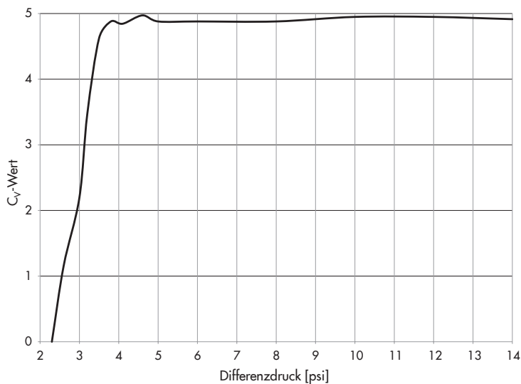
Bild 7-1: Ventilkennlinie und Durchflusstabelle für DN 15/NPS \frac{1}{2}
