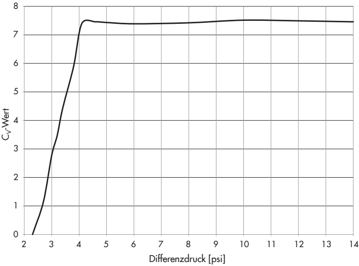
Bild 7-2: Ventilkennlinie und Durchflusstabelle für DN 20/NPS \frac{3}{4}
