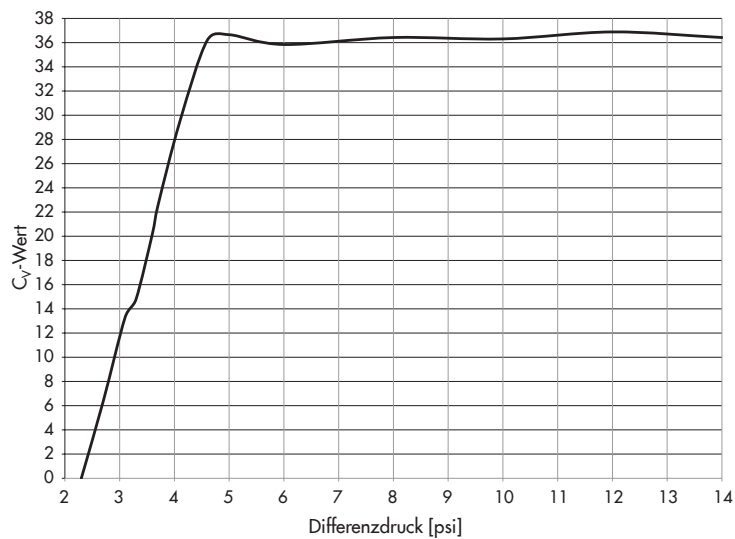
Bild 7-5: Ventilkennlinie und Durchflusstabelle für DN 50/NPS 2
