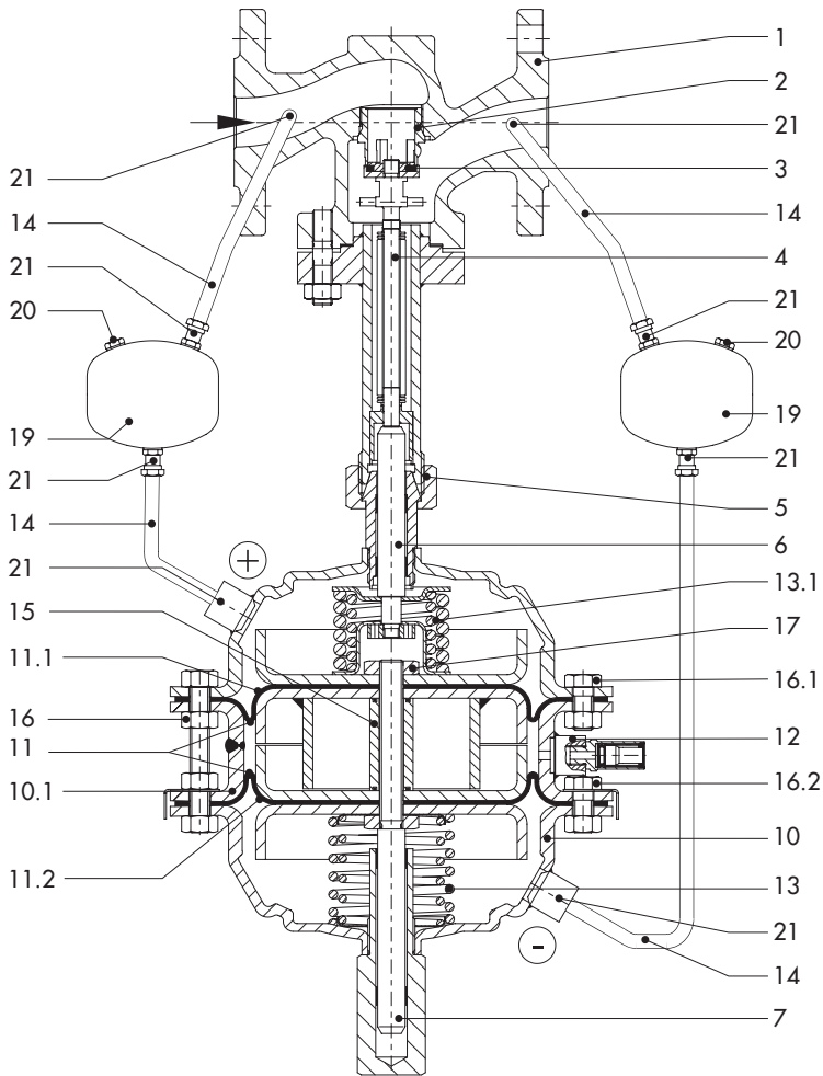
Bild 3-1: Aufbau und Wirkungsweise, Reglerdarstellung DN 15 bis 150/NPS ½ bis 6
