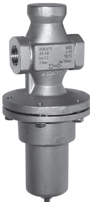
Muffengehäuse, Edelstahl
