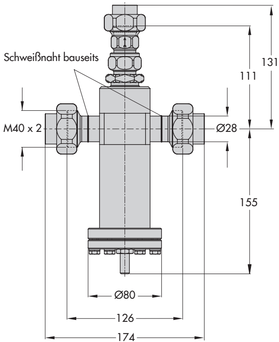
Bild 3-4: Abmessungen Ausführung CrNi-Stahl
