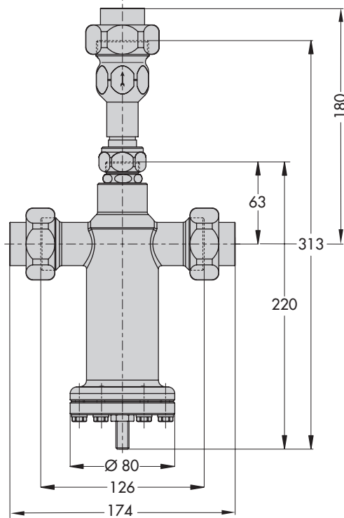
Bild 3-3: Abmessungen Standardausführung
