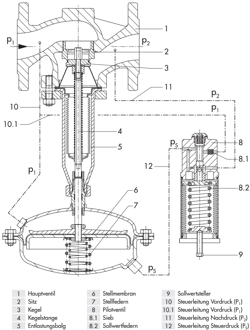
Bild 3-1: Aufbau und Wirkungsweise Typ 33-7
