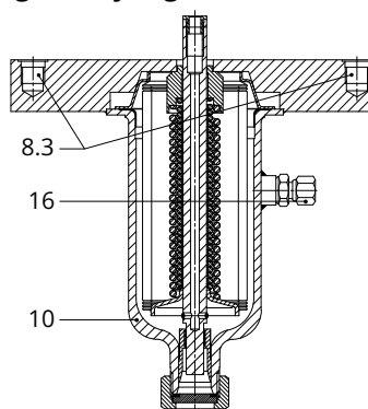
Balgaandrijving voor DN 65 tot 100
