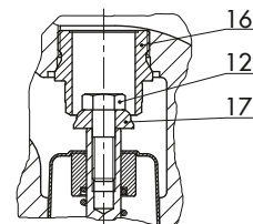
Standaarduitvoering DN 15 tot 25
