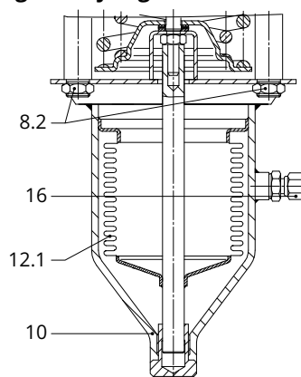
Balgaandrijving voor DN 15 tot 50
