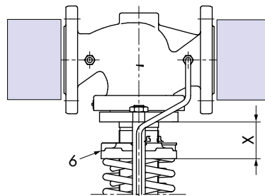
Afbeelding 12: Instelwaarde-voorinstelling via maat 'x'
