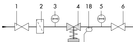
Afbeelding 10: Universele drukverlager van het type 41-23, schematisch inbouwvoorbeeld
