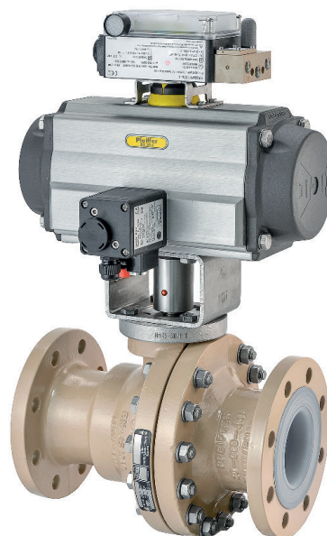
Fig. 2: Vanne à boisseau sphérique revêtue PFA BR 20b avec servomoteur rotatif BR 31a
