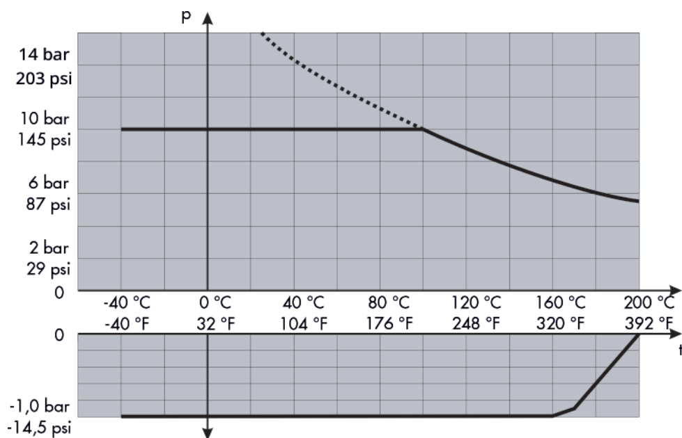
Bild 4: Pressure-temperature diagram
