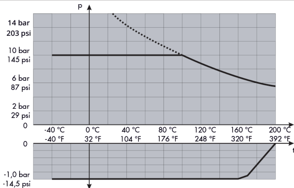
Bild 4: Druck-Temperatur Diagramm
