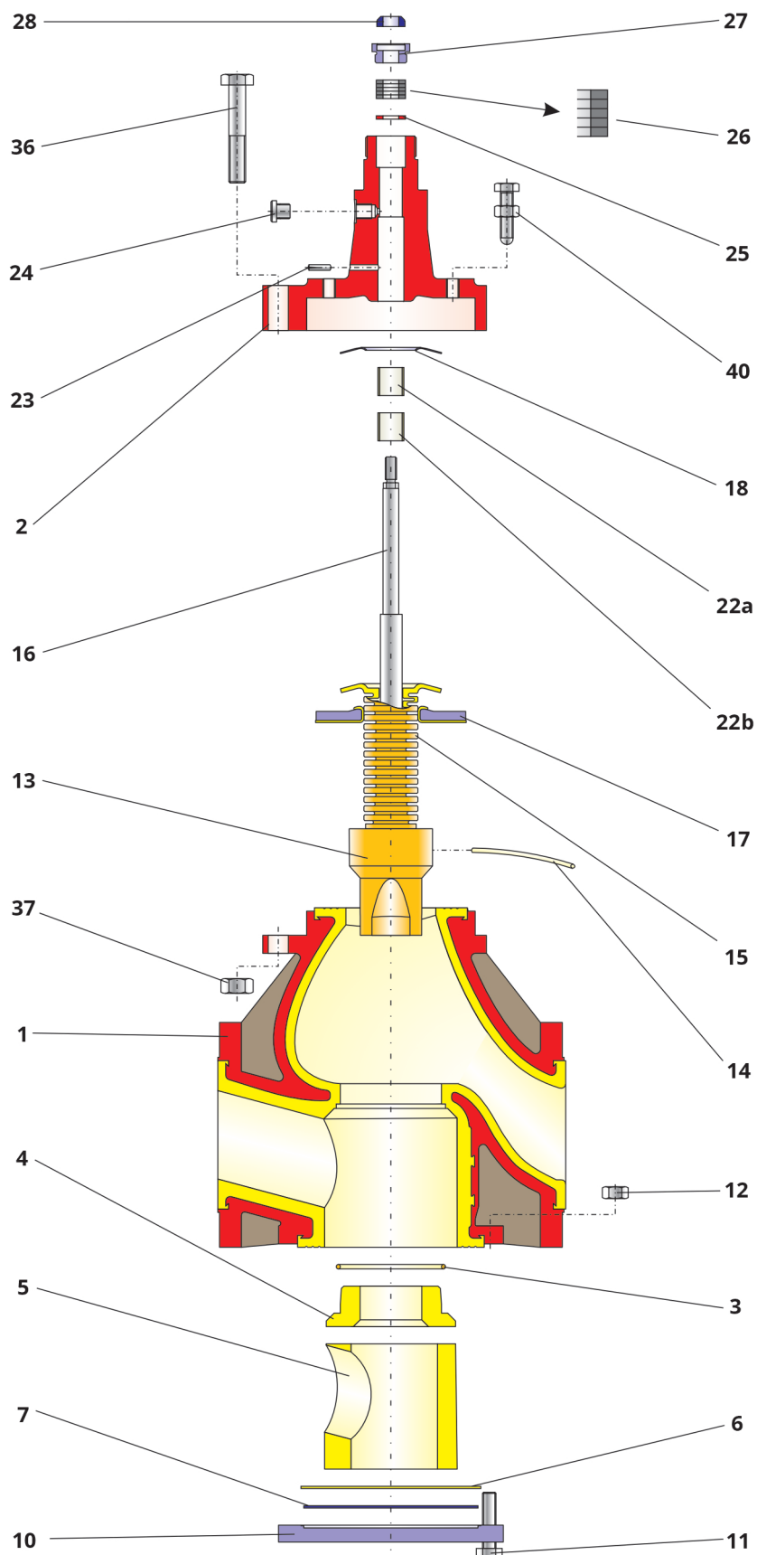
Bild 15-2: Explosionszeichnung des Ventils, DN 80 ... 150
