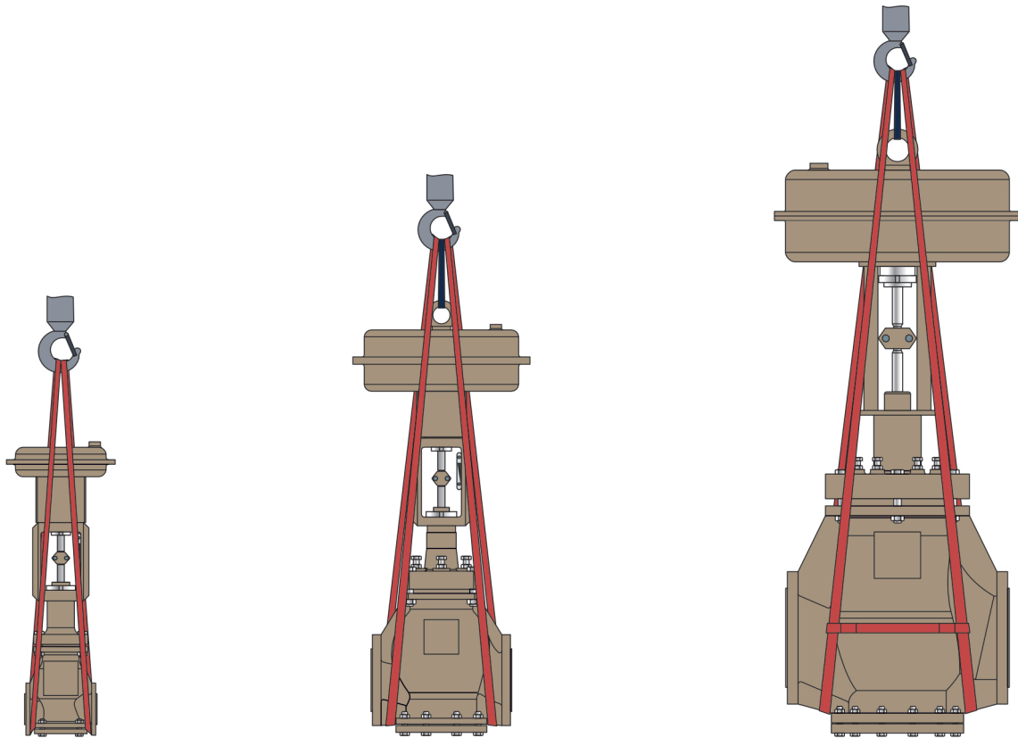
Hebeschlingen bei kleinen Nennweiten
