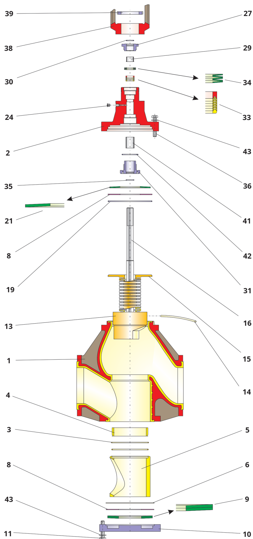
Bild 15-5: Explosionszeichnung des Ventils [G2], DN 200 und NPS8
