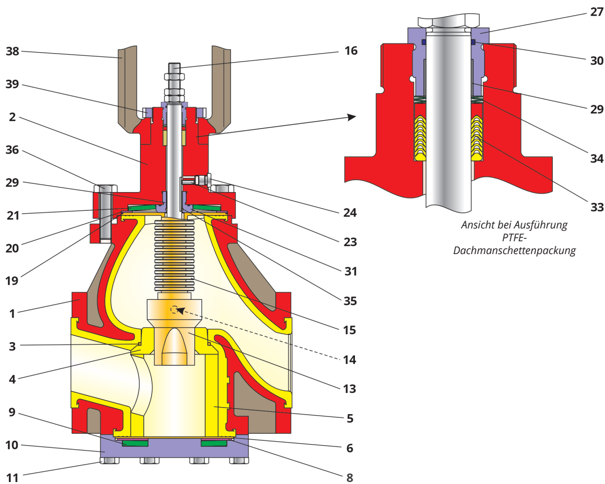
Bild 3-3: Schnitt durch ein Ventil [G2], DN 25 ... 80 und NPS1 ... 3
