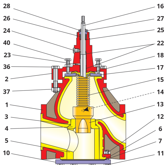
Schnitt durch ein Ventil DN 80 ... DN 150 / NPS4 ... NPS6
