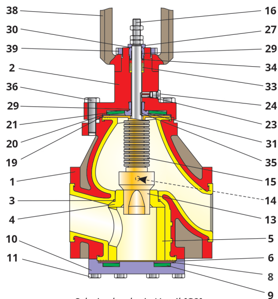
Schnitt durch ein Ventil [G2] DN 25 ... DN 80 / NPS1 ... NPS3
