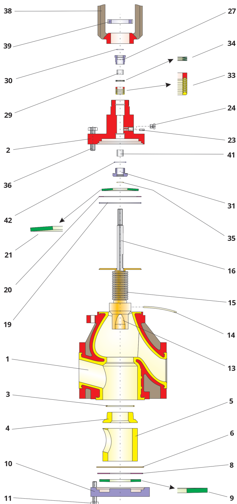
Bild 15-3: Explosionszeichnung des Ventils [G2], DN 25 ... 80 und NPS1 ... 3
