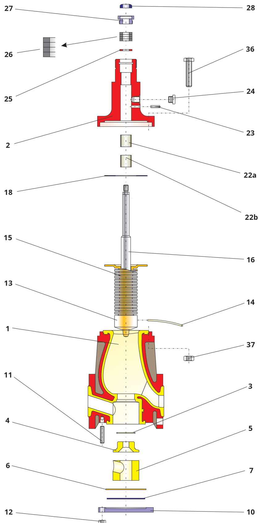
Bild 15-1: Explosionszeichnung des Ventils, DN 25 ... 50
